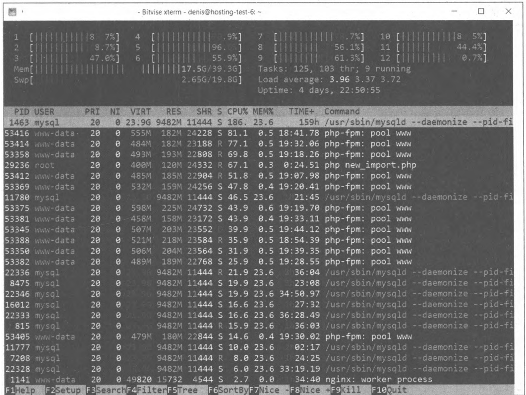
Рис. 11.21. Программа htop
